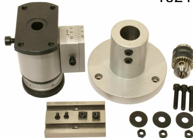
Umbausatz Fräsmaschine 10210
